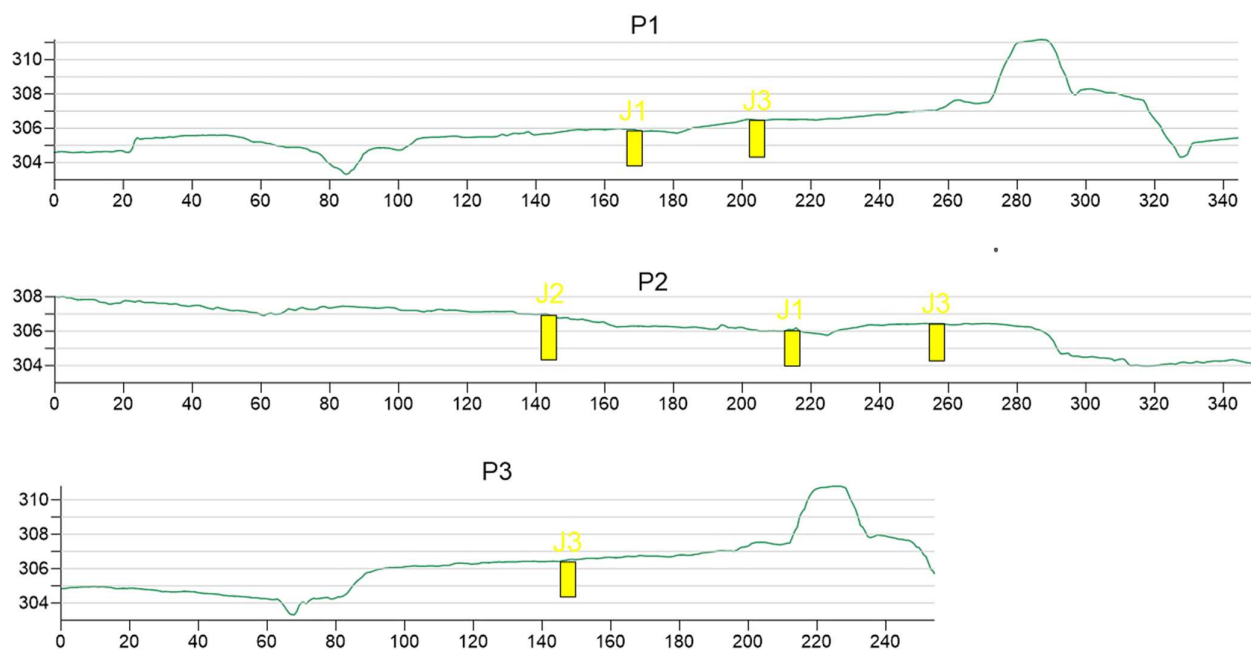
Slika 3: Prečni prerezi preko območja. Višina je 5x povečana. Prerez izdelan iz DMR posnetka (2014), zato so možna odstopanja. Sondažni jaški so prikazani. V območju J3 je vidno nasipavanje terena. Na terenu je debelina UN ca 0,7 m.
